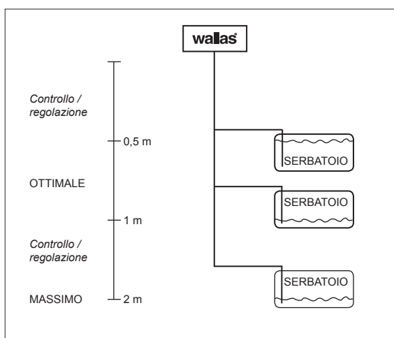
Posizione ottimale del serbatoio del carburante
