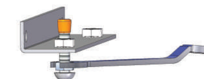
Tjockt bord
