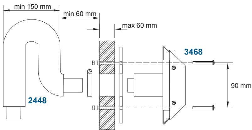
Allmän genomföring 3468 för förbränningsgaser och kylningsluft på båtens sidan. Installeringsutskärningen är \varnothing 45 mm och skruvhålen är 2 \times \varnothing 6 mm
