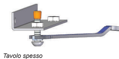
Agganciare i ferri di fissaggio alla stufa (3) utilizzando le viti (5).
