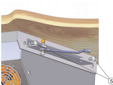
Kiinnitä kiinnitysraudat (3) liekeen ruuveilla (5)
